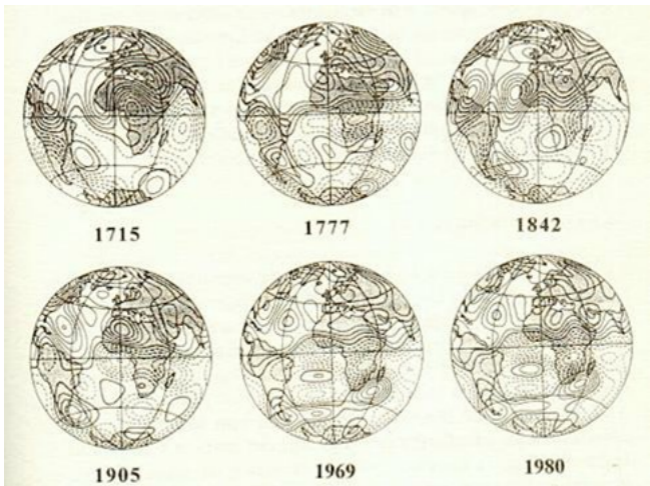
Figura 7.2. El cambiante campo magnético de la Tierra durante los últimos siglos. Los contornos de puntos
